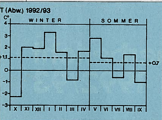
Diagramm 1: Die monatlichen und jahreszeitlichen Temperaturabweichungen von Bergstationen oberhalb 1500 m im Haushaltsjahr 1992/93.
