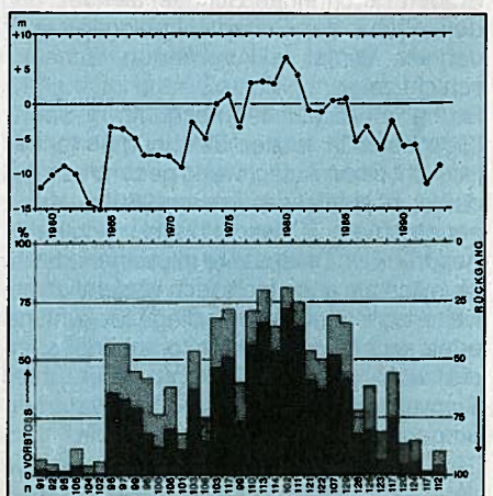
Diagramm 2: Die mittleren Längenänderungen der Ostalpengletscher (oben) und die Anteile vorstoßender (schwarz), stationärer (punktiert) und zurückschmelzender (weiß) Gletscherenden von der Anzahl (n) der beobachteten Gletscher.
