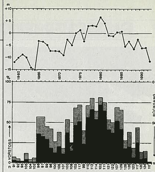
Diagramm 2: Die mittleren Längenänderungen der Ostalpengletscher (oben) und die Anteile vorstoßender (schwarz), stationärer (punktiert) und zurückgeschmelzender (weiß) Gletscherenden von der Anzahl (n) der beobachteten Gletscher.
